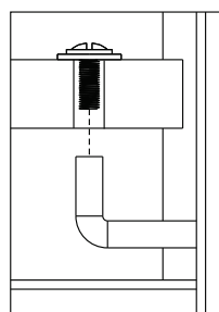
Fixação do estrado lado direito
